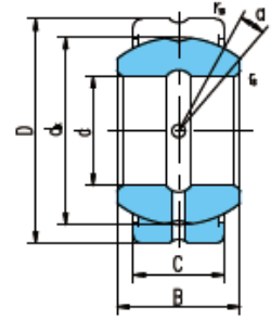
GEZ...ES-2RS
